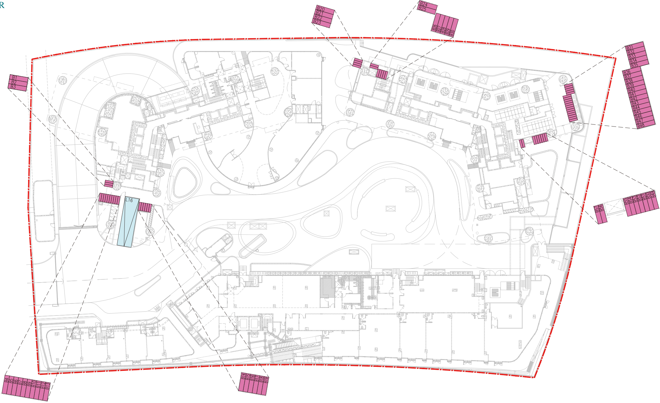
Location, Numbers, Dimensions and Area of Parking Spaces on Ground Floor 地下的停車位的位置、數目、尺寸及面積
